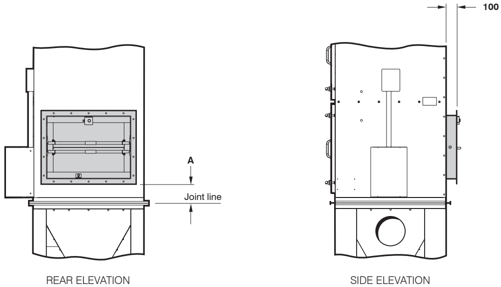
POSITION OF OPTIONAL EXPLOSION RELIEF FLANGE UMA 153 illustrated
